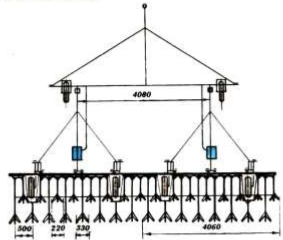
РИС. 131. СХЕМА РАССТАНОВКИ ГРЯДИЛЕЙ И ПРУЖИННЫХ РЫХЛИТЕЛЬНЫХ ЛАП
