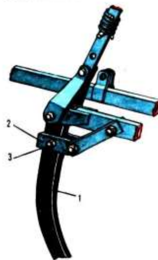
1 — стойка; 2 — кронштейн; 3 — стопорный винт
