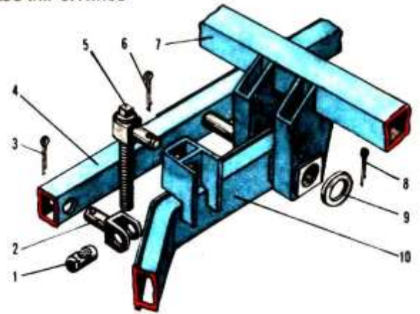
1 — гайка винта; 2 — цапфа; 3, 6, 8 — шплинты; 4 — кронштейны колеса; 5 — винт; 7 — брус рамы; 9 — шайба; 10 — брус сннца
